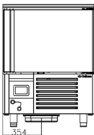
ALZADO
