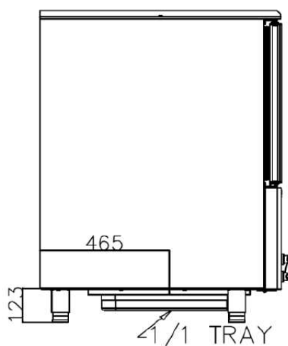
PERFIL
