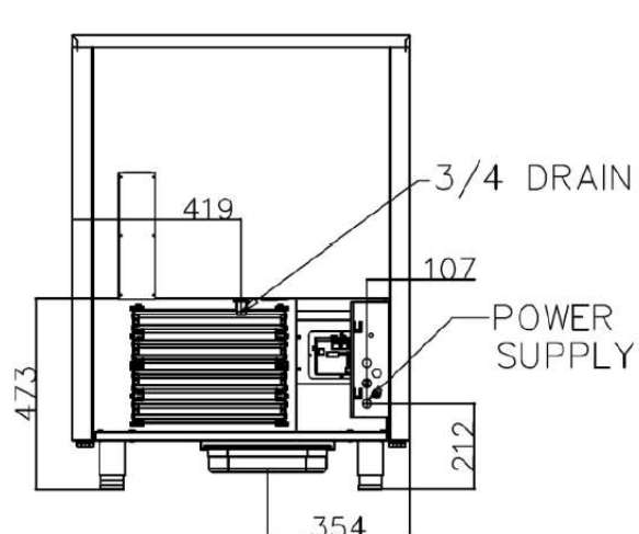
TRASERA
